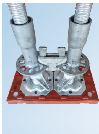
Appui avec collier double à clavette
