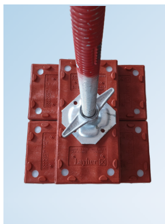
Empilement des cales sans risque de glissement
