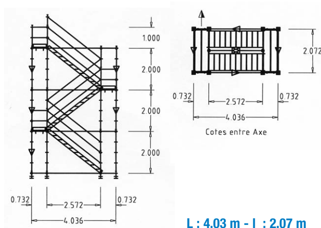
Modèle C Tour à 8 pieds avec volées en acier de 2,57 m x 0,75 m de large
