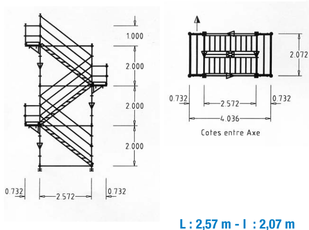
Modèle A Tour à 4 pieds avec volées en acier de 2,57 m x 0,75 m de large
