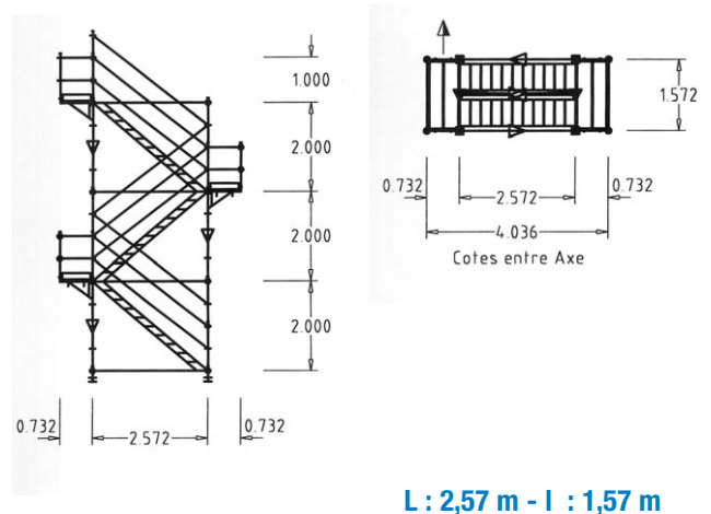
Modèle B Tour à 4 pieds avec volées en aluminium de 2,57 m x 0,58 m de large
