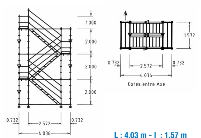
Modèle D Tour à 8 pieds avec volées en aluminium de 2,57 m x 0,58 m de large
