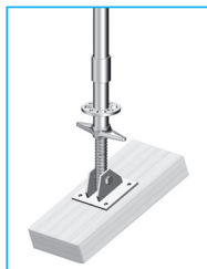
Avec un madrier de 8 x 22 x 50 cm
