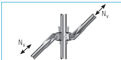
Effort axial sur diagonale LW (daN)
