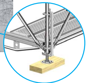
Fixation éventuelle des madriers sous les socles par vissage ou cloutage
